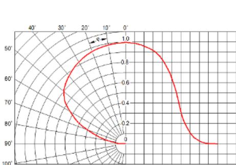
Рисунок 4 Типы КСС
