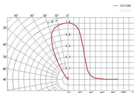
Рисунок 4 Типы КСС
