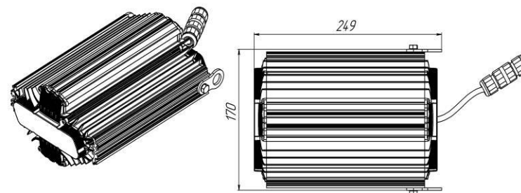
Рисунок 1 Светильник «L-lego 30» Подвесное крепление.
