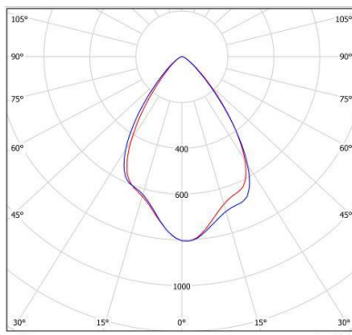
Исполнение «Г33»
