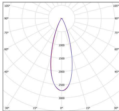
Исполнение «Г33»
