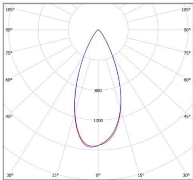
Исполнение «К12»
