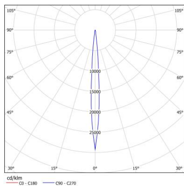
Исполнение «К8»
