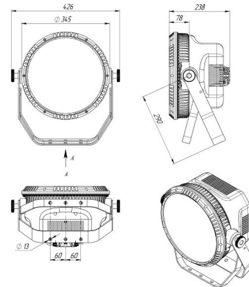
Рисунок 1 Габаритные размеры светильника «L-banner 600»
