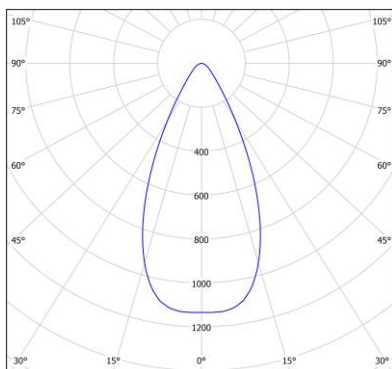
Исполнение «К12»
